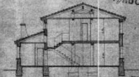
Sección
