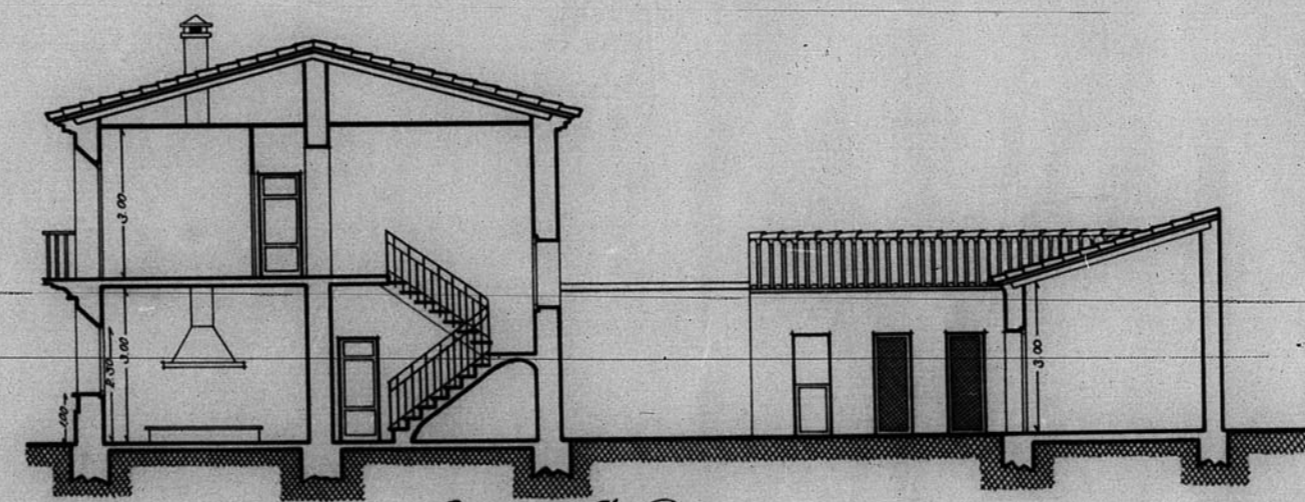
Sección A.B.
