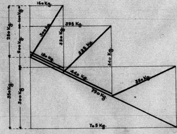
Escala de fuerza 10 m.m. = 100 Kg.
