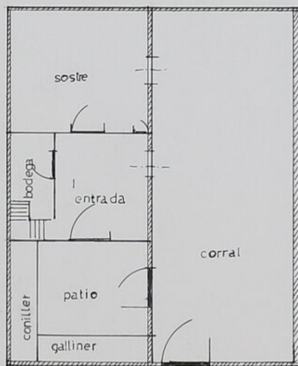
planta baixa
