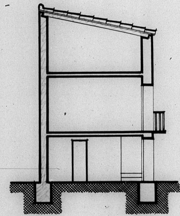
SECCION A-B.
