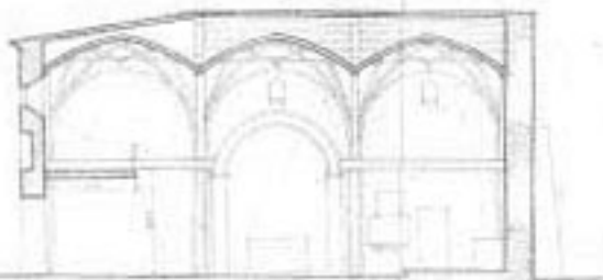
Sección C-D
