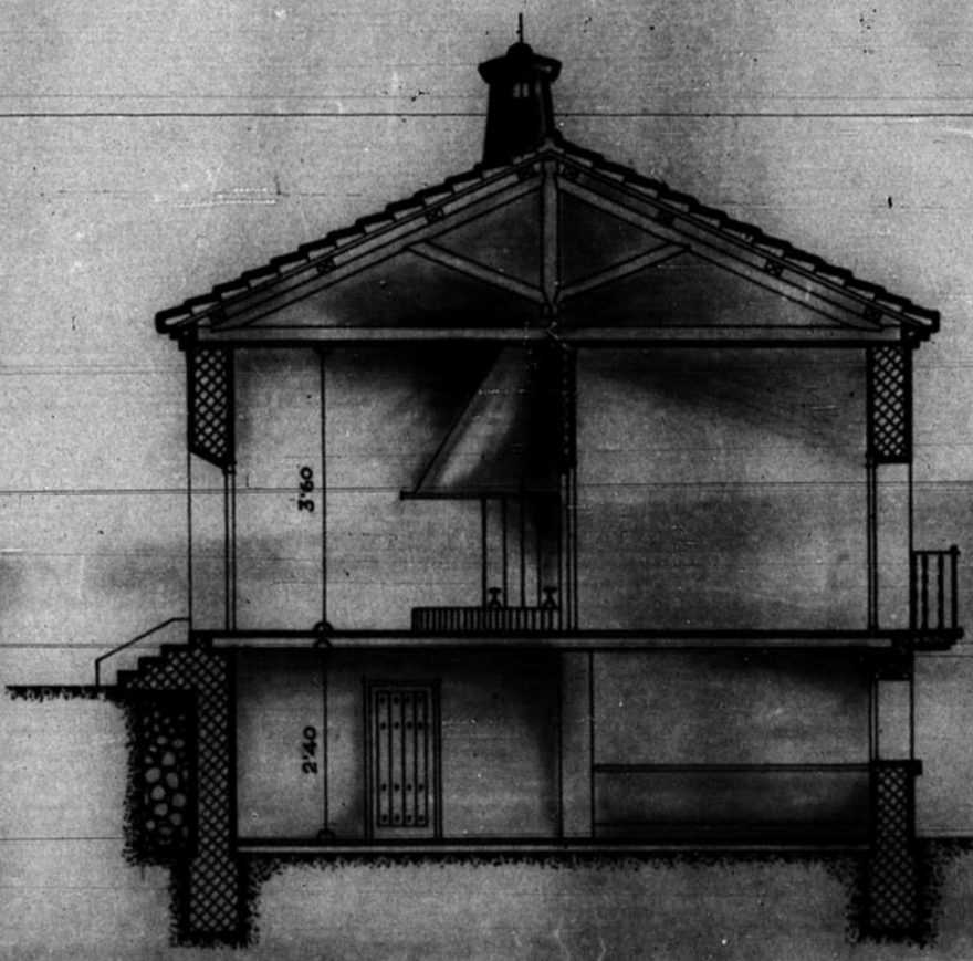
— Sección A-B —
