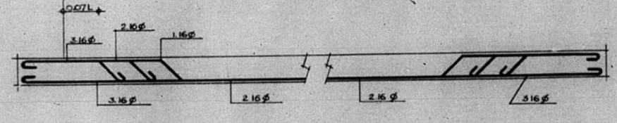
DETALLE LONGITUDINAL
