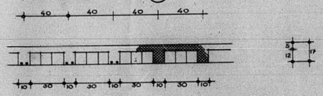
FORJADO TIPO d
