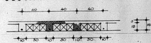
DETALLES LONGITUDINALES DEL NERVIO
