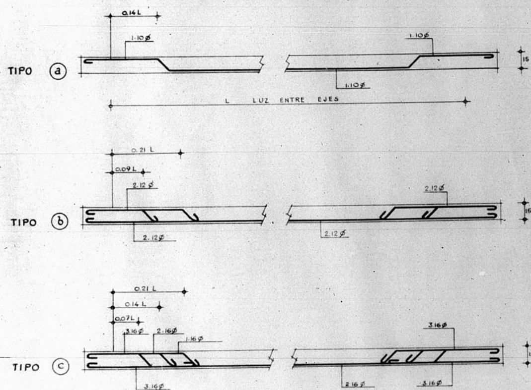
DETALLES LONGITUDINALES DEL NERVIO
