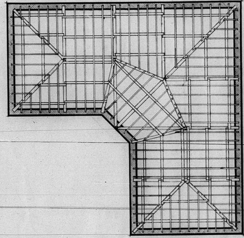
Entramado de cubierta
