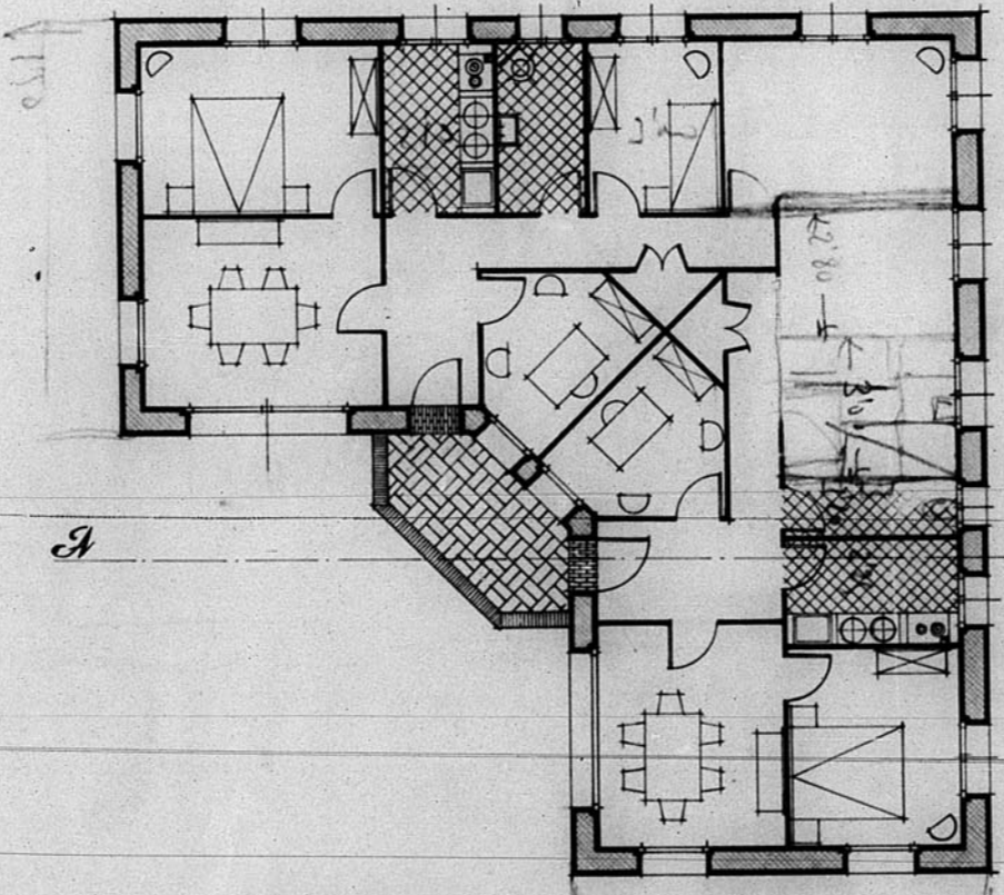
Planta
